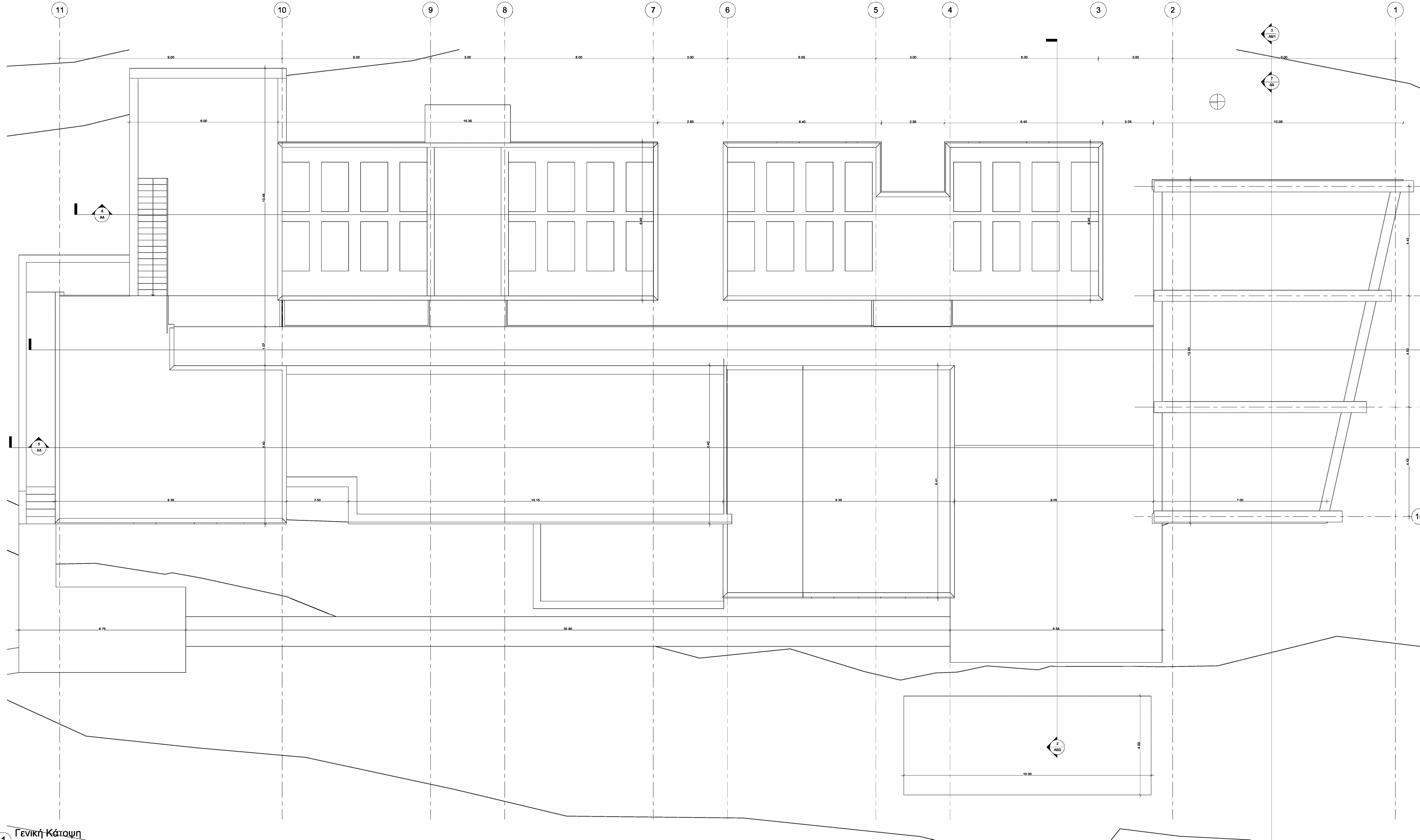
1 Γενική Κάτοψη 1 : 50
